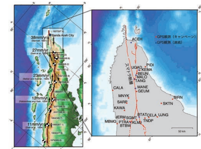
(左) スマトラ島における過去の地震活動とスマトラ断層のすべりの速度 (右) スマトラ断層を横断する形で構築された、AGNeSSの観測点分布
