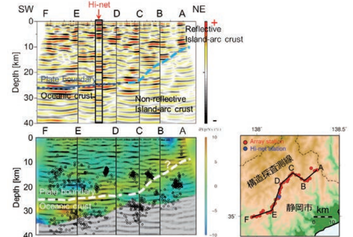
レーバ関数(上)とトモグラフィ(下)から求めた静岡県中部、南アルプス南端部のフィリピン海プレート沈み込み構造
