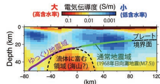
日向灘の地下における電気伝導度分布
