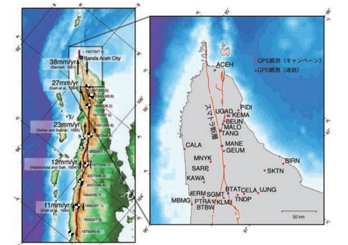
(左) スマトラ島における過去の地震活動とスマトラ断層のずれの速度 (右) スマトラ断層を横断する形で構築された、AGNeSSの観測点分布
