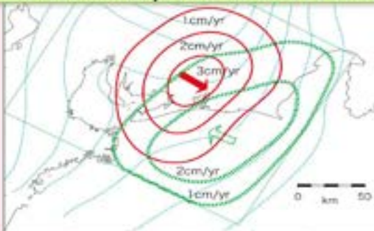
データ解析・モデリング Data analysis and modeling
