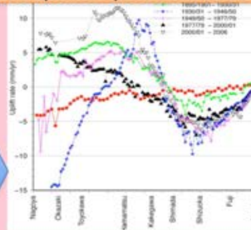
地震発生サイクルと発生予測 Earthquake cycle and forecast
